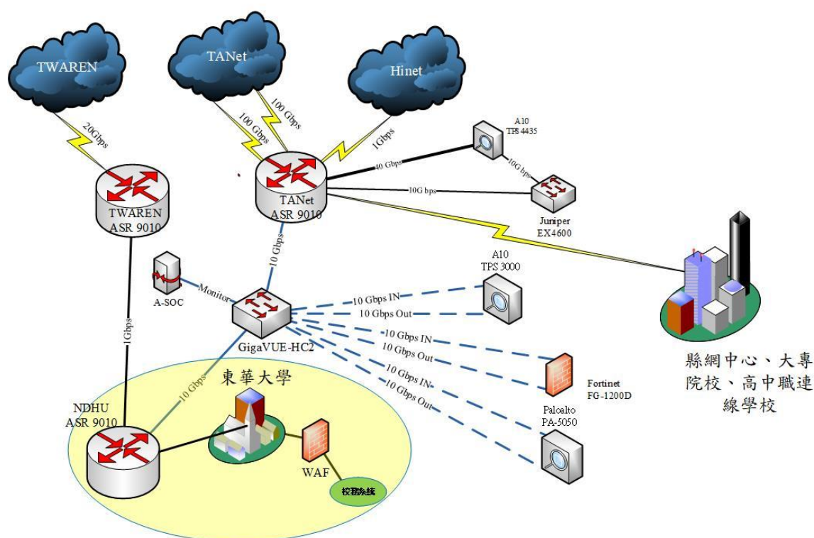
圖十、資安防護網路架構
